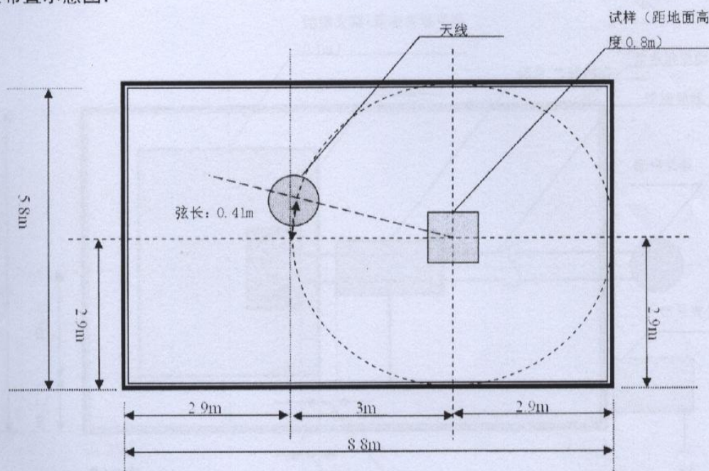
试验布置示意图:
